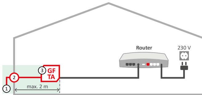
Abbildung 1: Beschreibung Glasfaser-Hausanschluss
